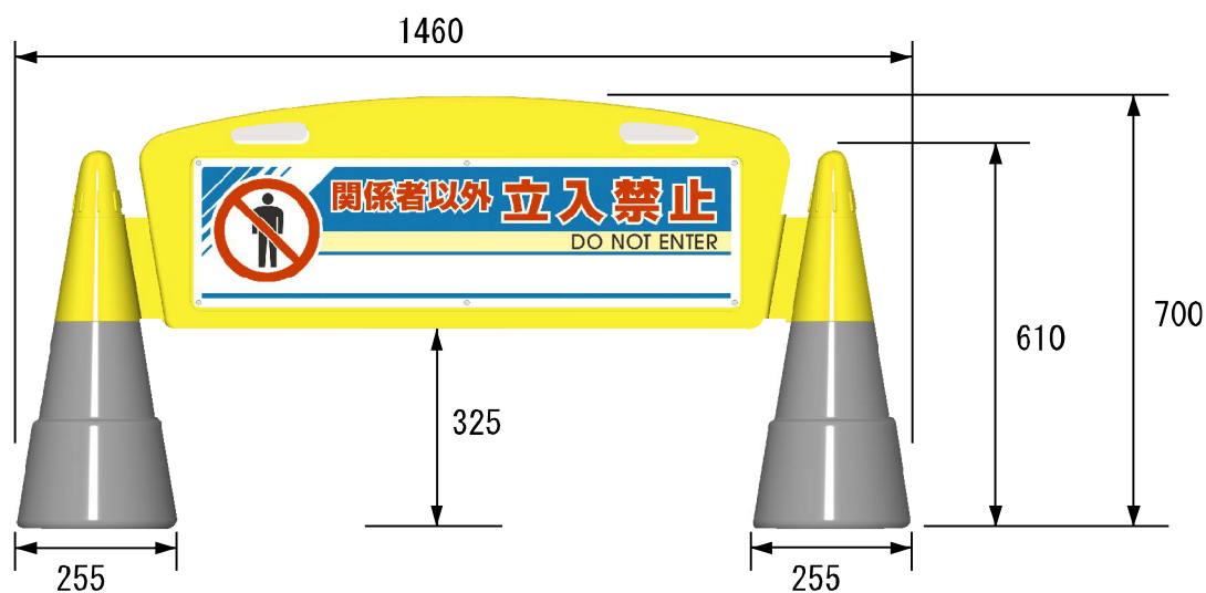
■ 寸法図 (mm)
